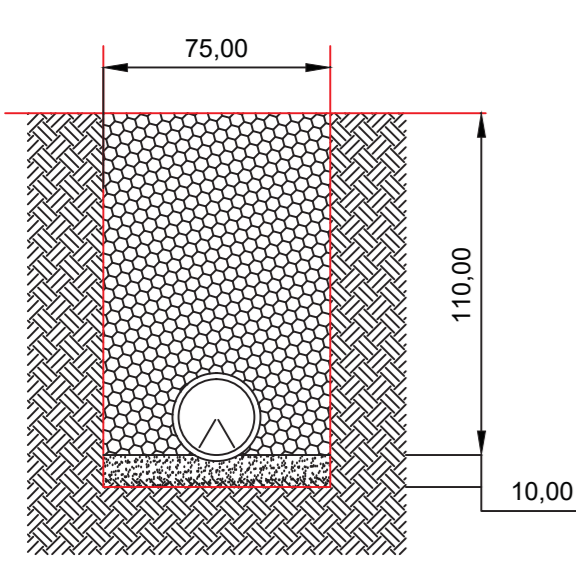
TUBAZIONE diam 250 / 200 mm
